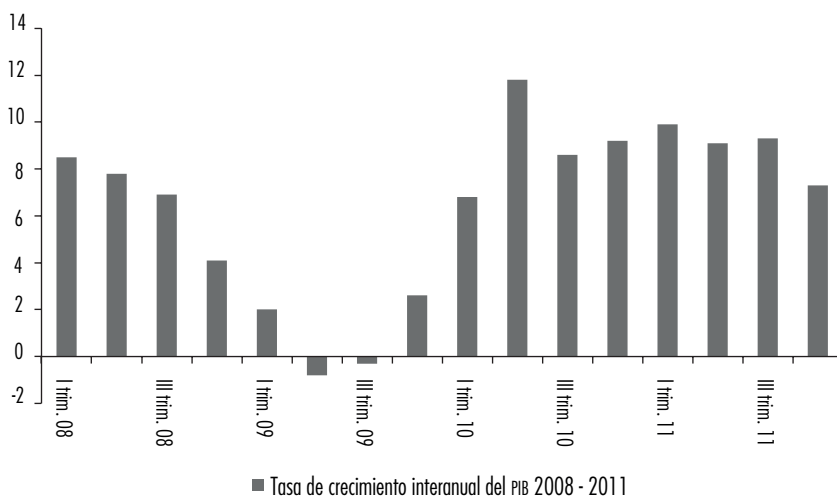
Gráfica 2. Tasa de crecimiento interanual del PIB a precios constantes
